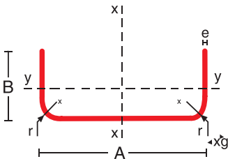
PGU PERFIL U
