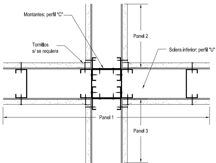
ENCUENTRO DE PANELES EN CRUZ
