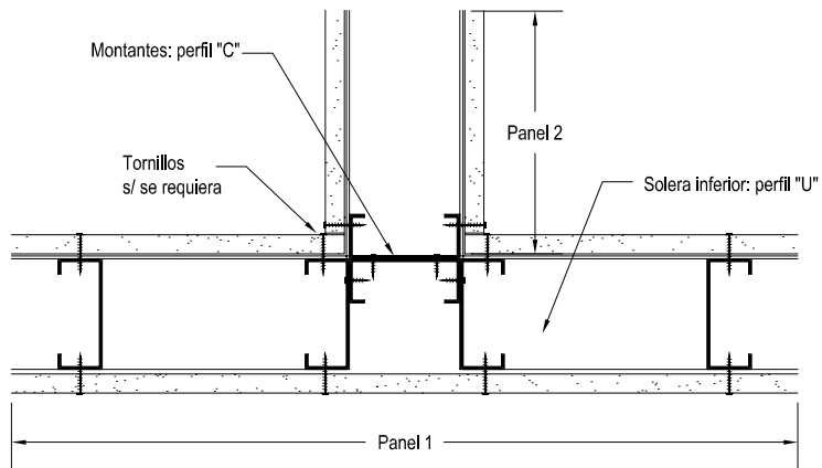
ENCUENTRO DE PANELES EN "T"
