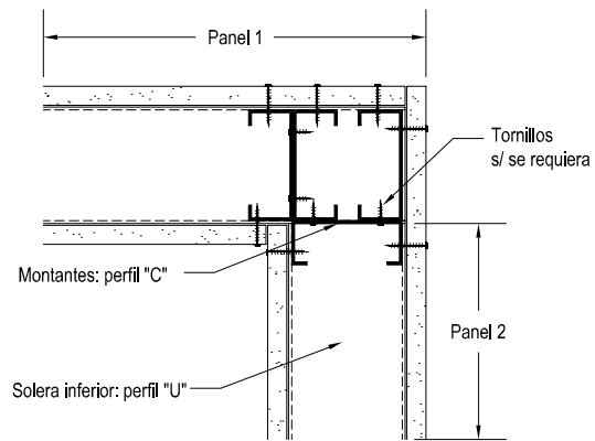
ENCUENTRO DE ESQUINA
